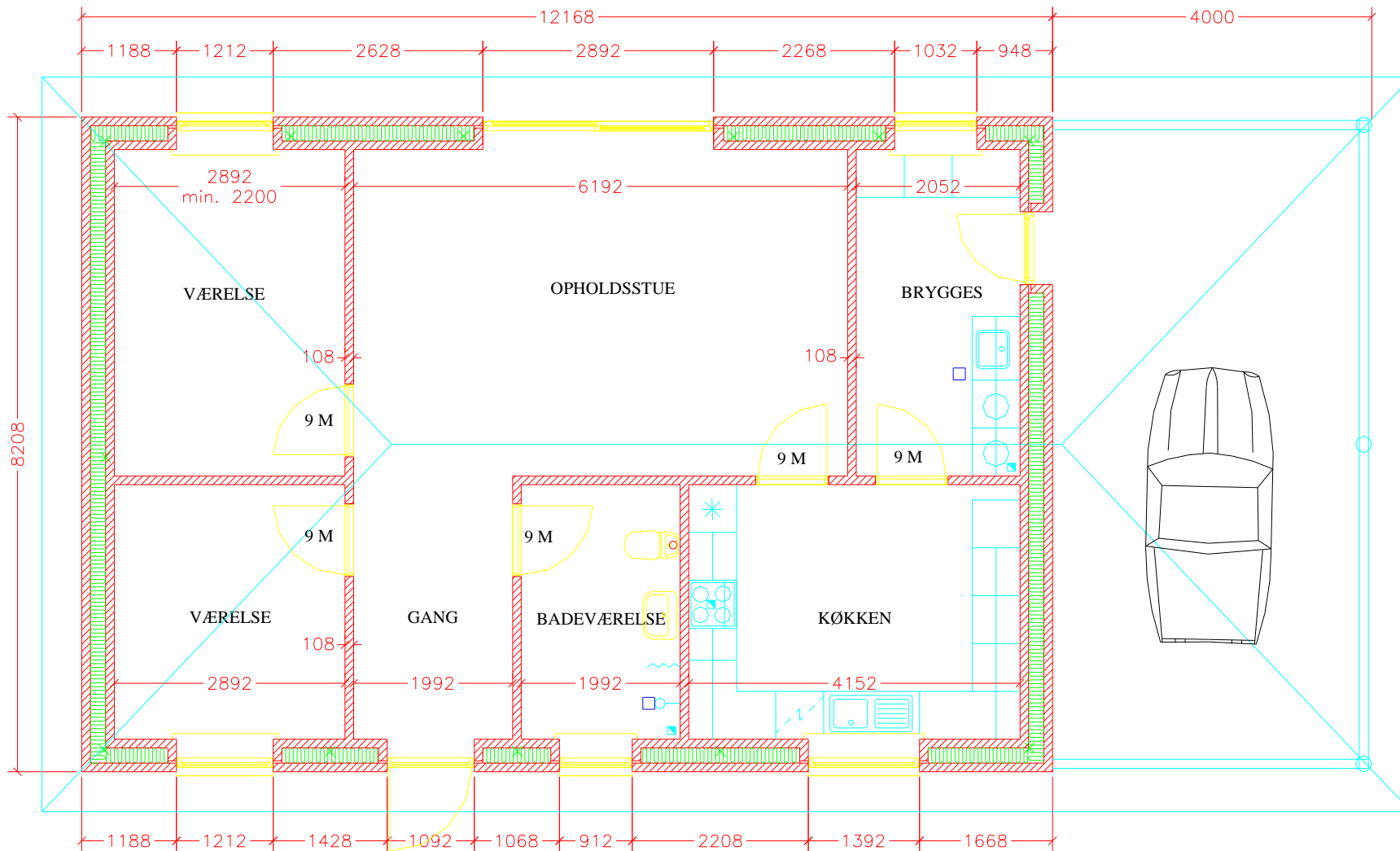
Grundplan 1:100
